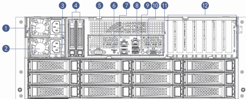
3.5 × 36 后面板示意图
