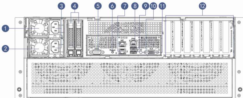
3.5 × 24 后面板示意图
