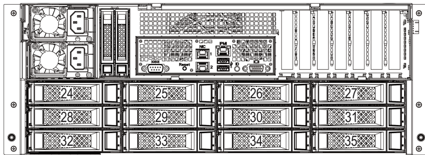
3.5 × 36 后面板硬盘顺序图
