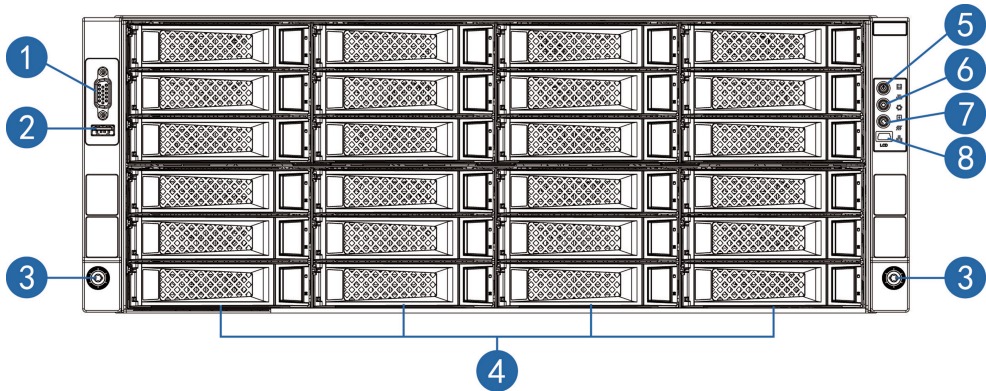
前面板示意图
