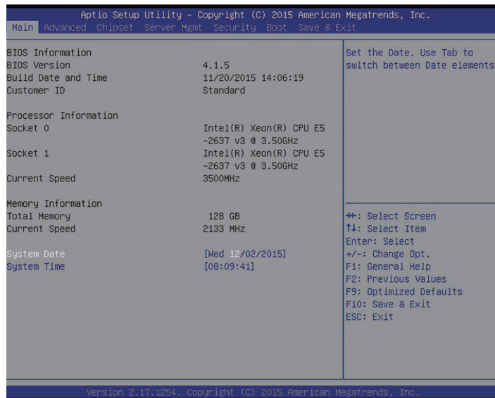
Main 菜单界面说明表
